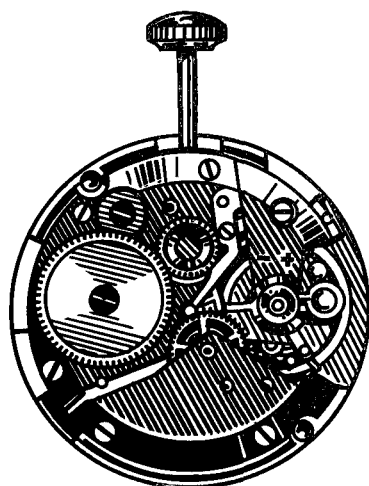
Ø 24 мм, H = 4,35 мм
