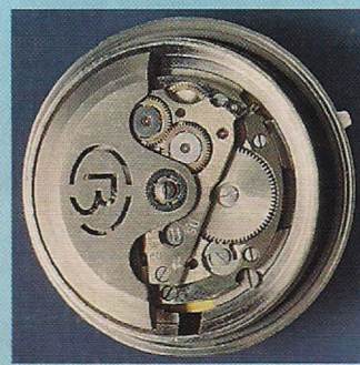
Das Automatik-Uhrwerk des Modells «KGB OPERATIONAL».
